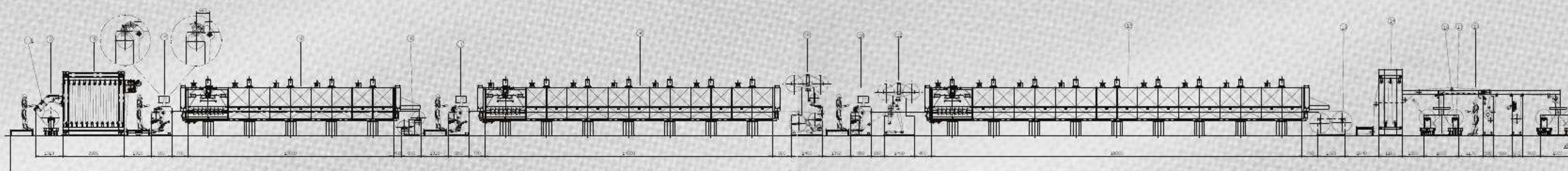
Triple Head Knitted Fabric Transfer Coating Head (3 Kafalı Örme Kumaş Kaplama Transfer Hattı)
